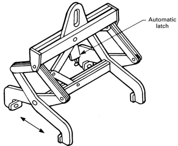
(d) Automatic Slab Tong (Four Point)
