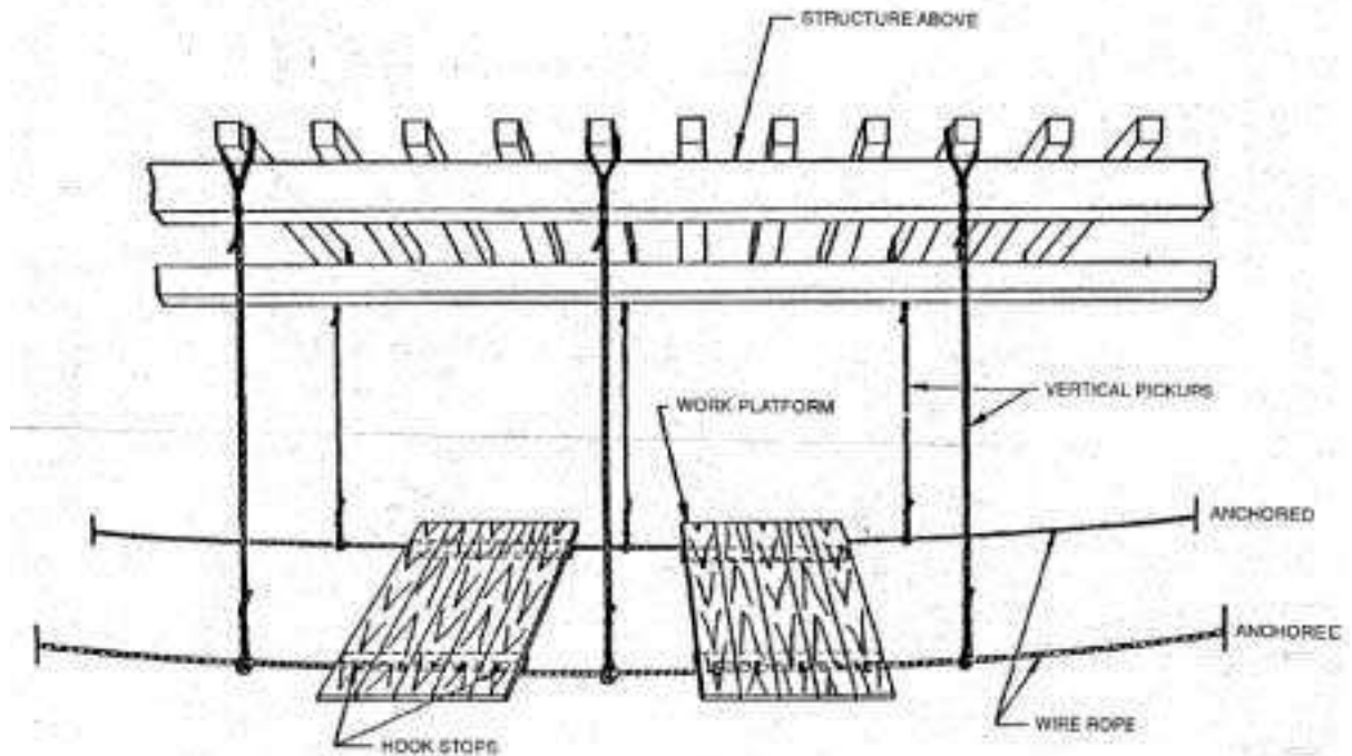
الشكل. السقالات السلسلية
